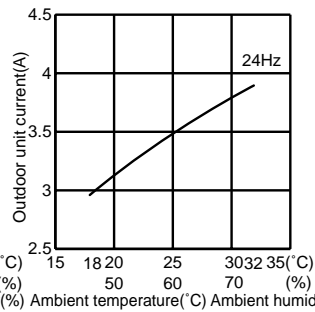
MUZ-A26YV - [E1]
