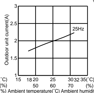
MUZ-A18YV - [E1] (Indoor unit : MSZ-A18YV - [E1])
