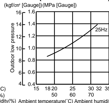
MUZ-A18YV - [E1] (Indoor unit : MCFZ-A18WV - [E1])
