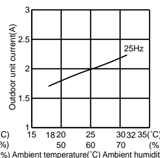
MUZ-A18YV - [E1] (Indoor unit : MCFZ-A18WV - [E1])
