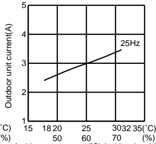
MUZ-A26YV - [E1]
