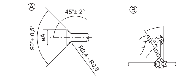
(A) Dimensioni di taglio per raccordo a cartella (B) Coppia di serraggio del dado a cartella
